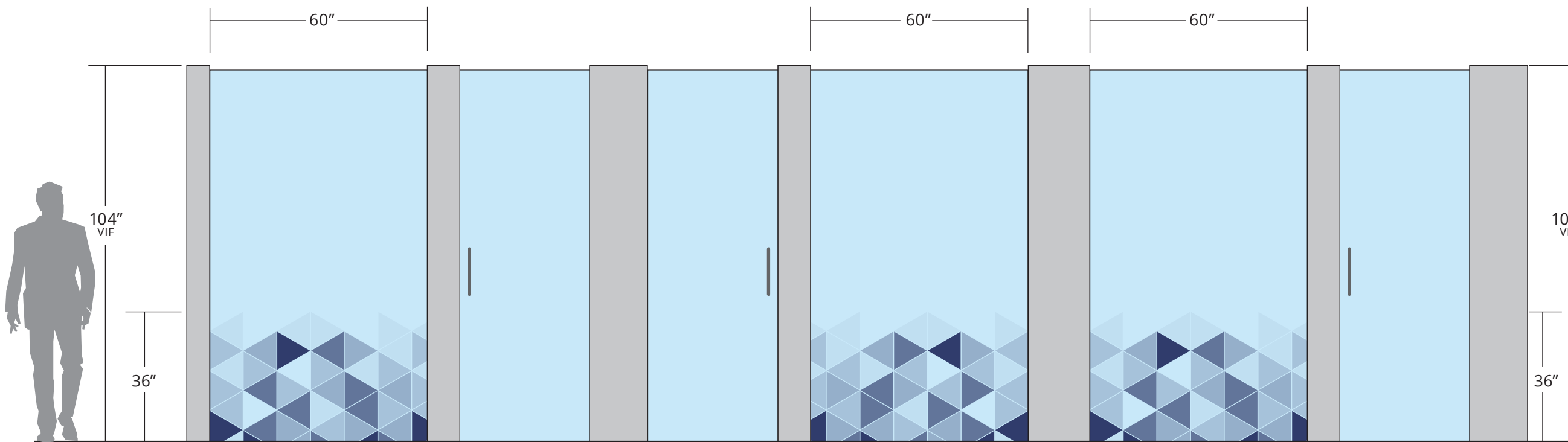
③ OFFICE #3 scale: 3/8" = 1'-0"
